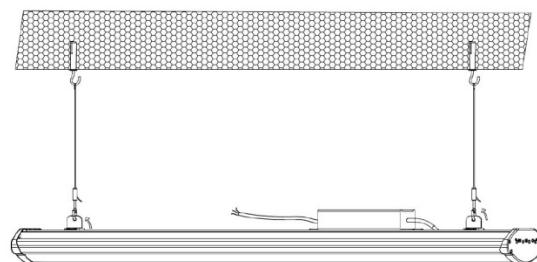
Montagebeispiel (Seilsystem im Lieferumfang)
